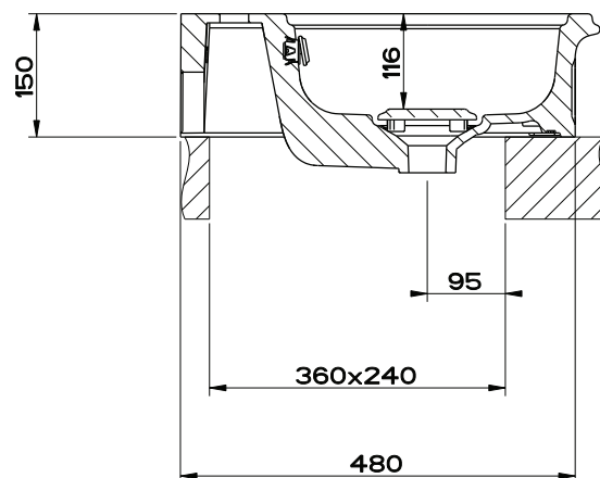
SEZIONE B-B
